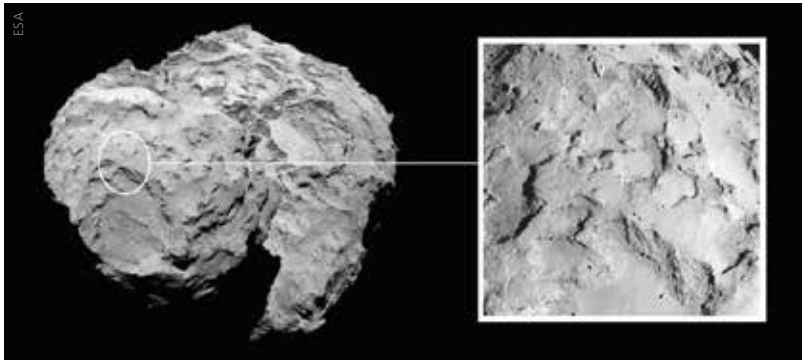
Die fünf hier markierten möglichen Landestellen kamen bei einem Meeting am 23. und 24. August 2014 in die Endauswahl. Sie sind in einem Bild dargestellt, das von der OSIRIS-Kamera am 16. August 2014 aus einer Entfernung von 100 Kilometern gemacht wurde.
