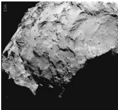
Nahaufnahme der geplanten Landestelle von Philae.
